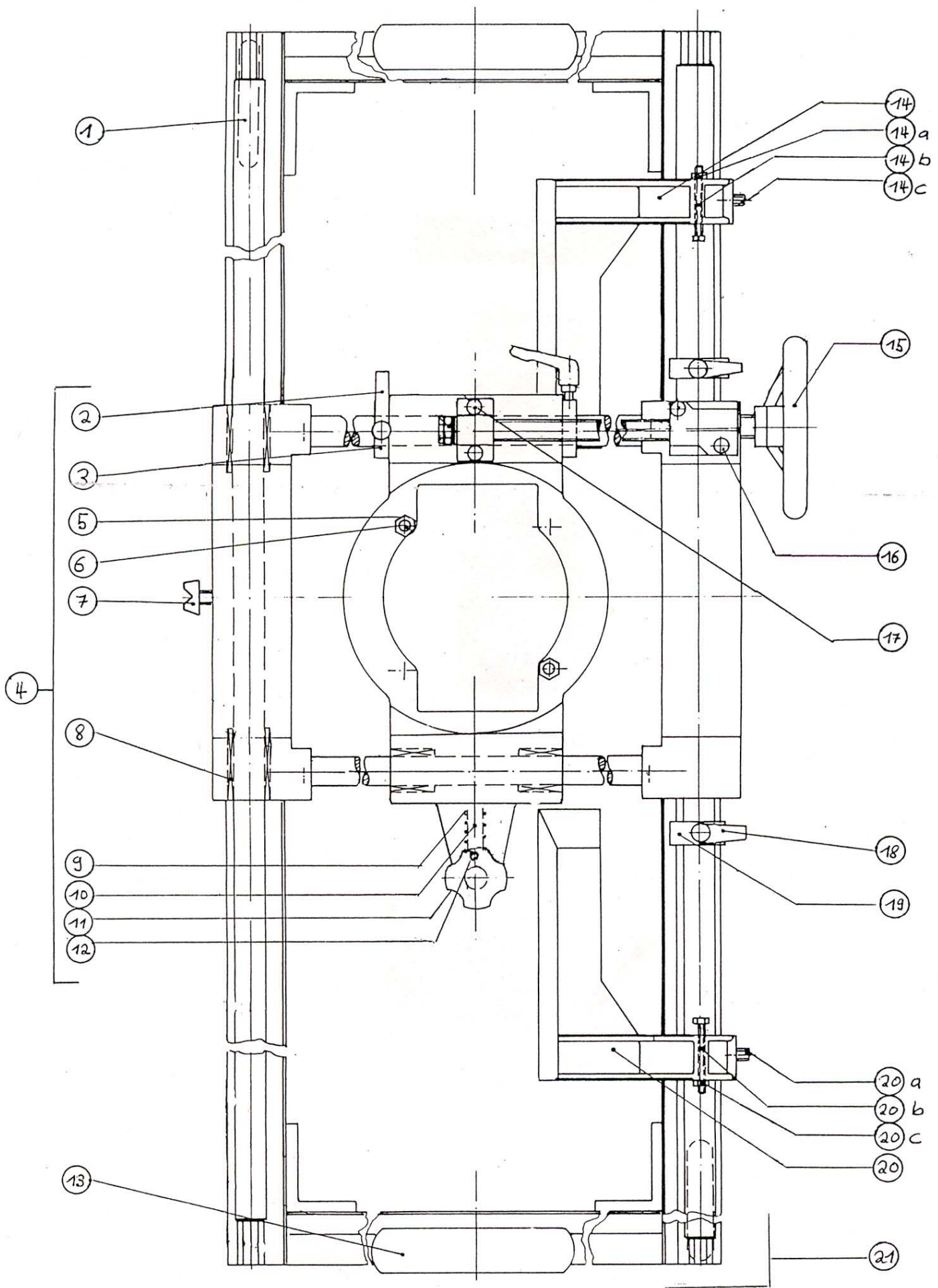
Treppenwangen-Fräsergerät TW4-2
